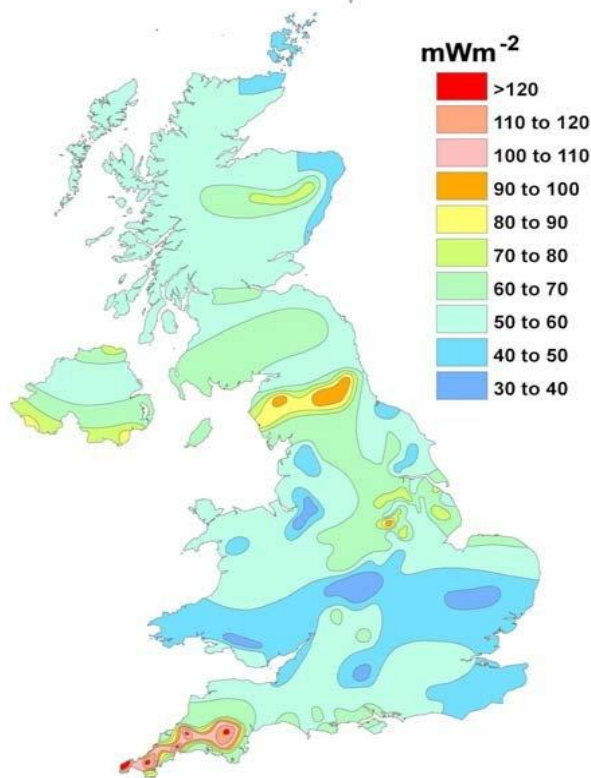
UK heat flow map (Busby, 2010)
